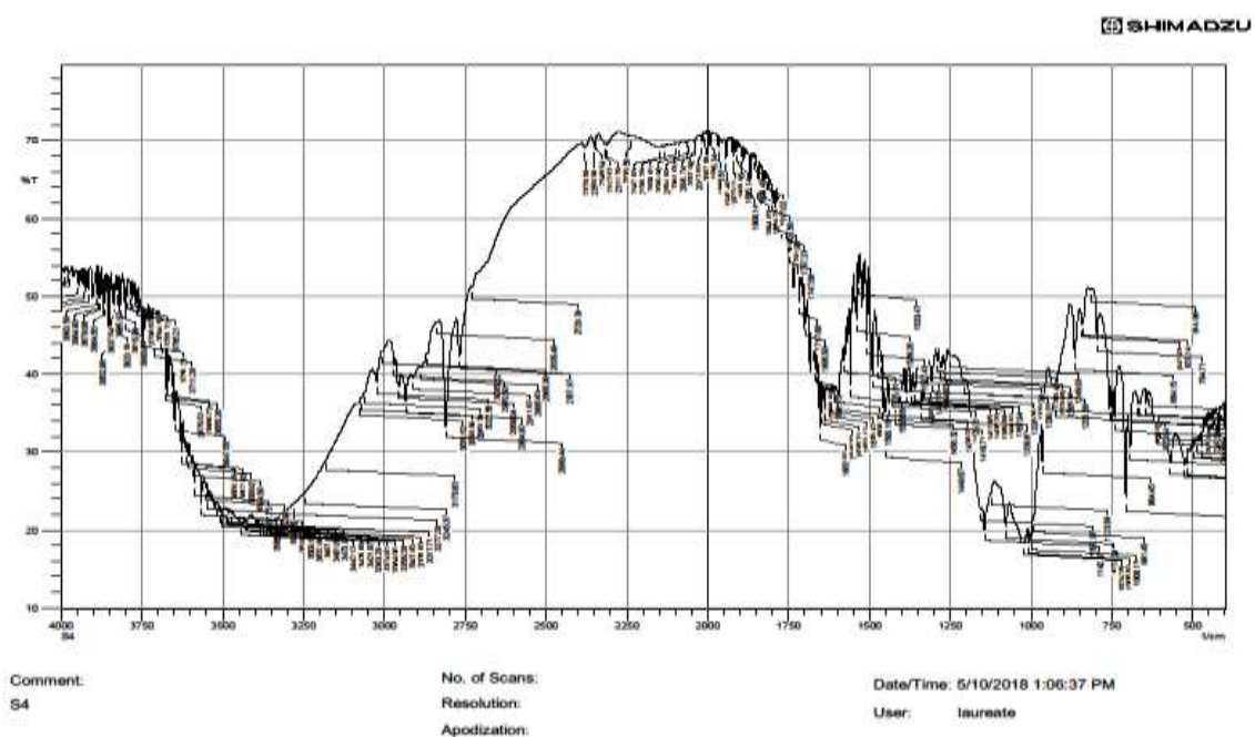
Figure 13 FTIR Spectrum of CNZ + SA
